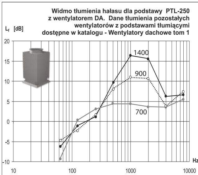
Wartości tłumienia hałasu w dB podstawy PTL-250 dla poszczególnych częstotliwości Hz, dla poszczególnych obrotów wentylatorów o średnicy wlotu Ø250.
