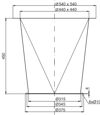
Przyłącze kołnierzone pod podstawę tłumiącą
