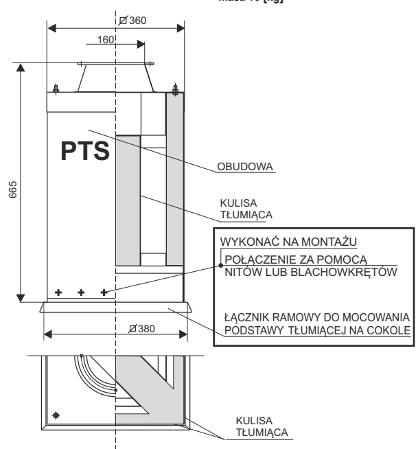
PODSTAWA TŁUMIĄCA PTS-160 masa 16 [kg]
