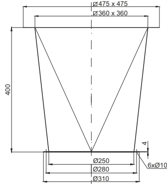
Przyłącze kołnierzone pod podstawę tłumiącą
