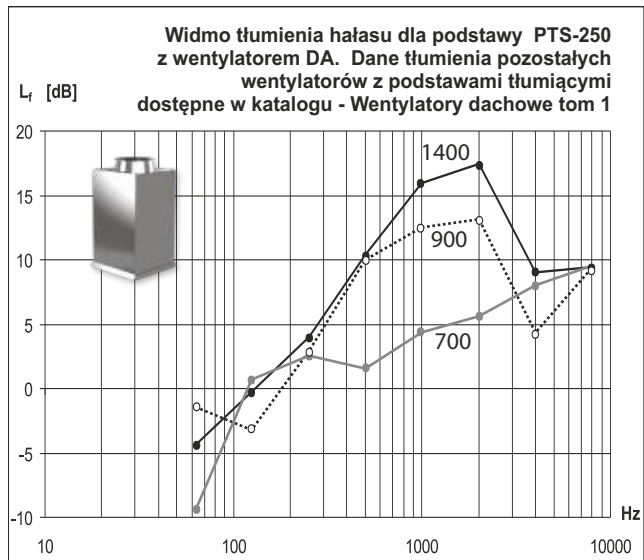
Wartości tłumienia hałasu w dB podstawy PTS-250 dla poszczególnych częstotliwości Hz, dla poszczególnych obrotów wentylatorów o średnicy wlotu Ø250.
