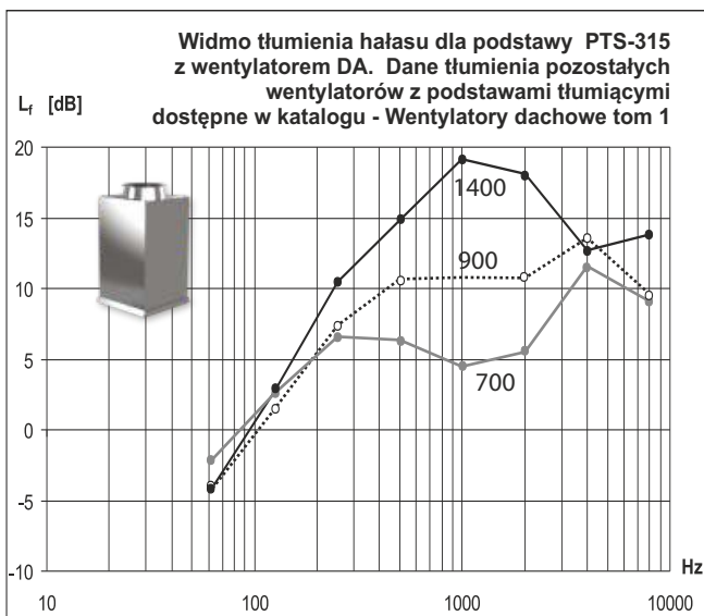
Wartości tłumienia hałasu w dB podstawy PTS-315 dla poszczególnych częstotliwości Hz, dla poszczególnych obrotów wentylatorów o średnicy wlotu Ø315.
