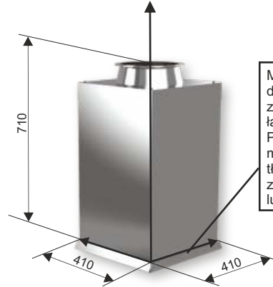
PODSTAWA TŁUMIĄCA PTS-200 masa 25 [kg]
