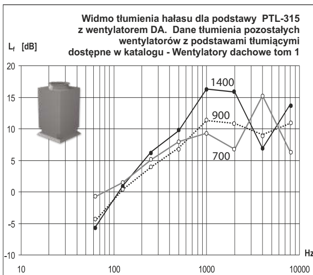
Wartości tłumienia hałasu w dB podstawy PTL-315 dla poszczególnych częstotliwości Hz, dla poszczególnych obrotów wentylatorów o średnicy wlotu Ø315.
