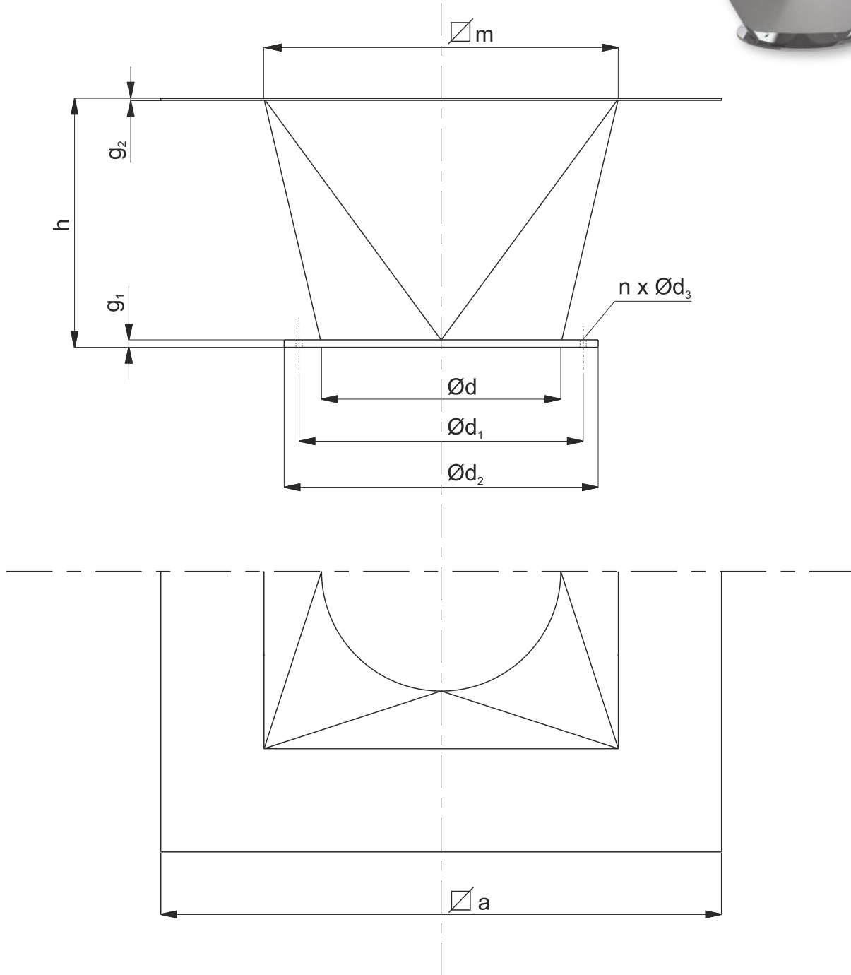
PRZYŁĄCZE KOŁNIERZOWE DLA PTL
